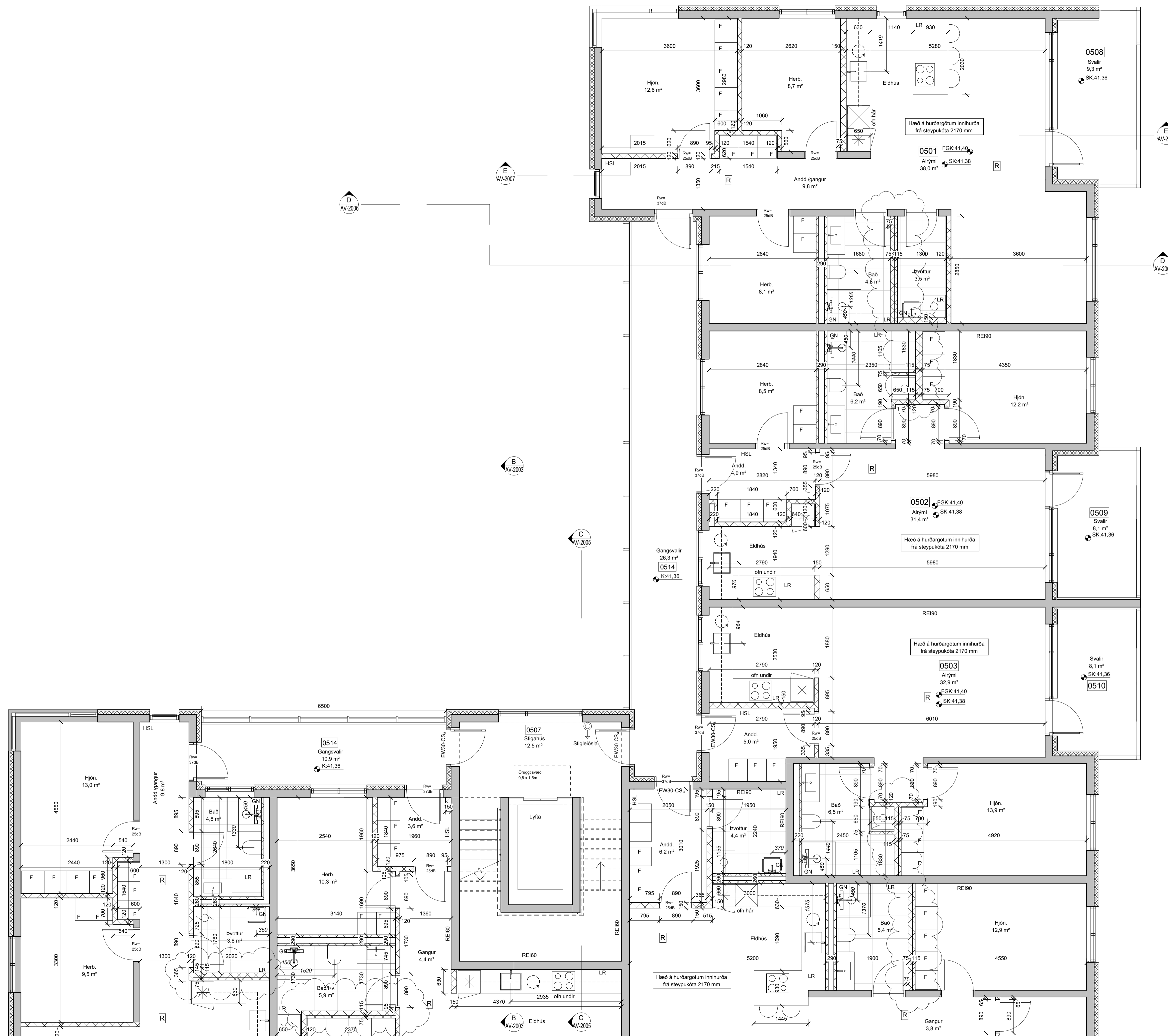
5. HÆÐ - VERKTEIKNING - A mkv: 1 : 50
