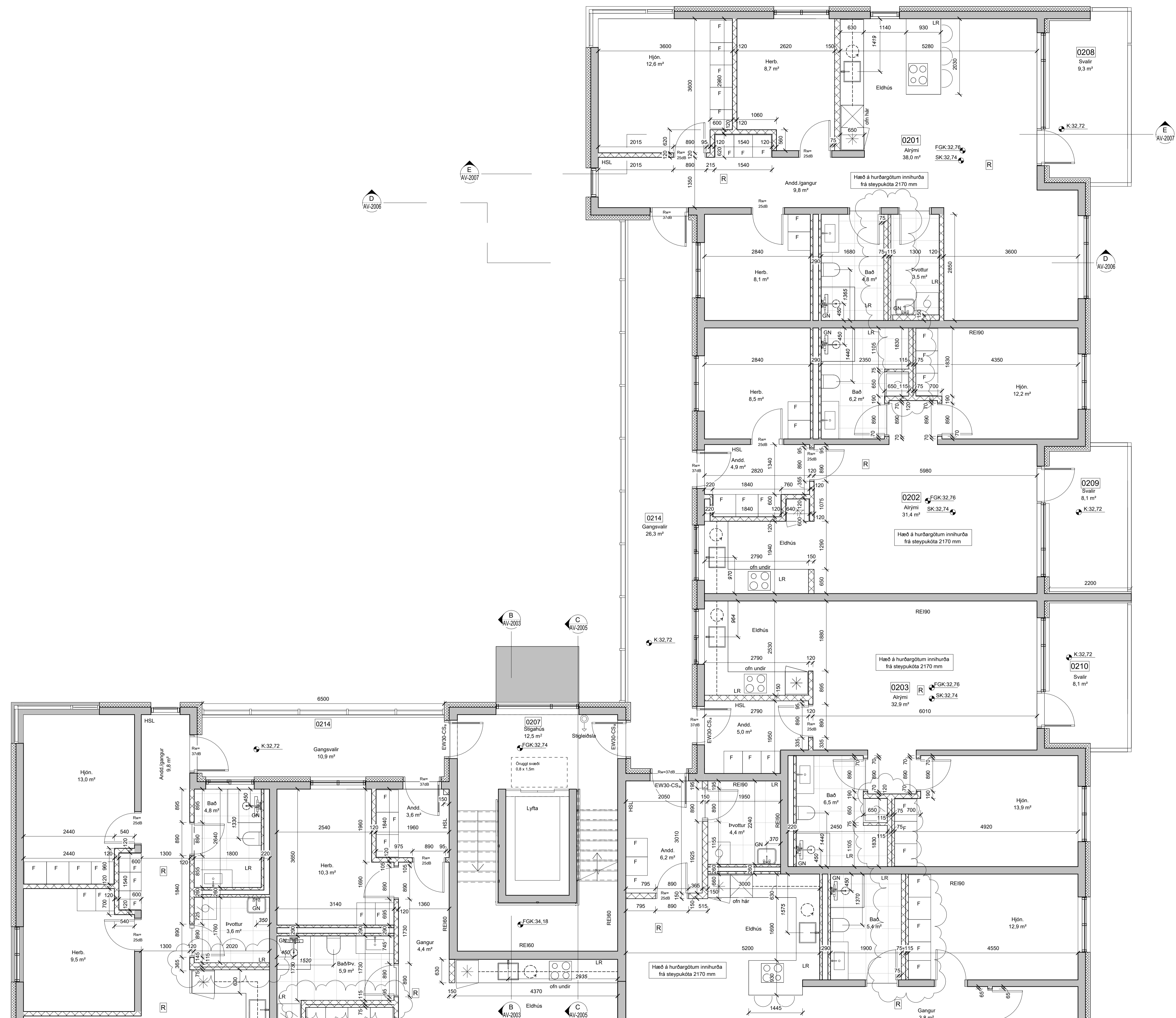
2. HÆÐ - VERKTEIKNING - A mkv: 1 : 50
