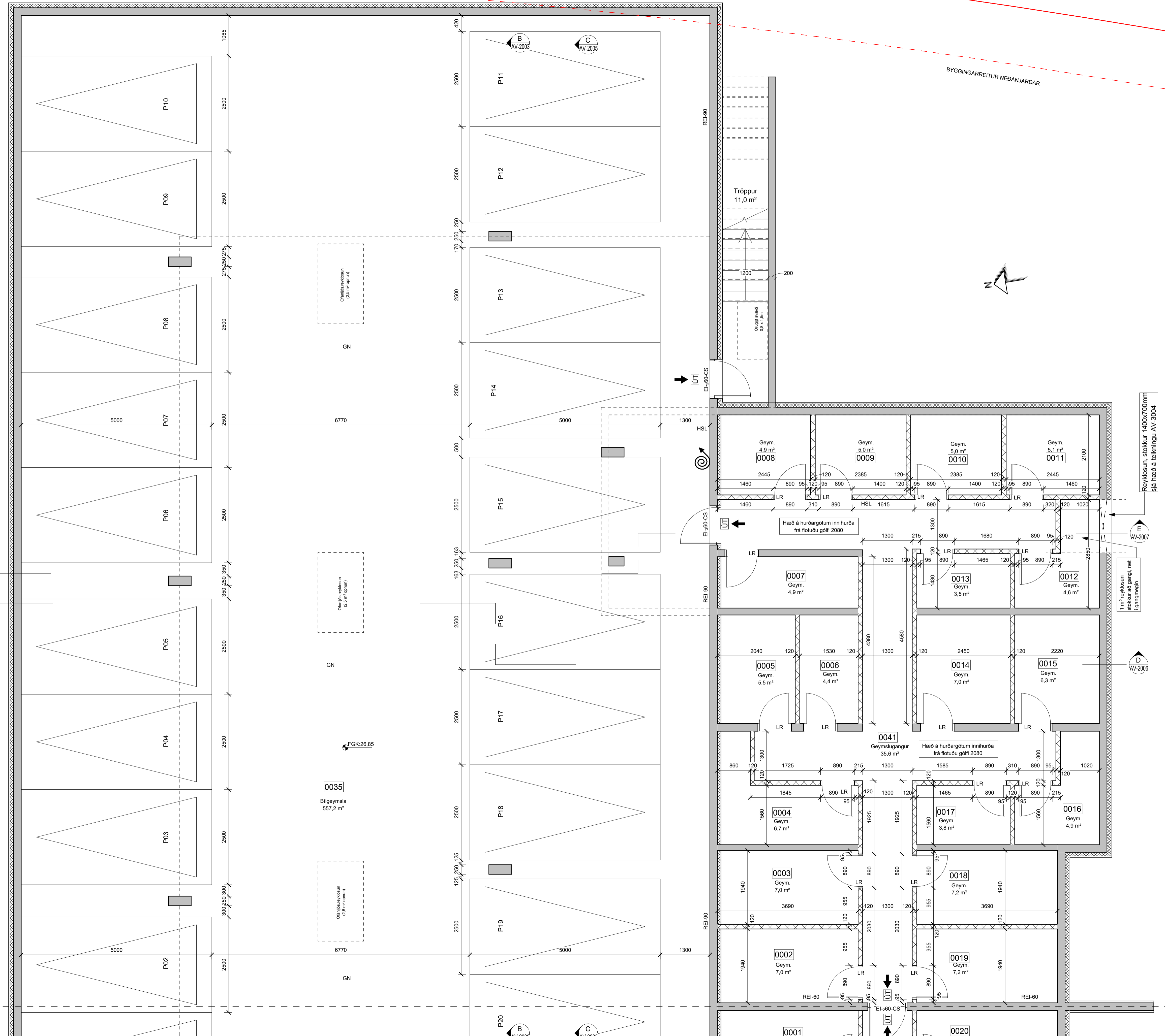
0. KJALLARI - VERKTEIKNING - A mkv: 1 : 50
